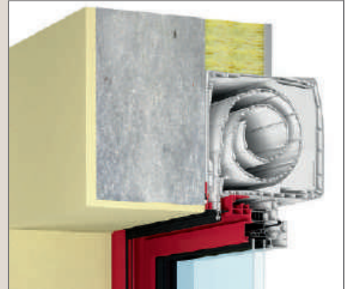
Le bloc-baie Classic
