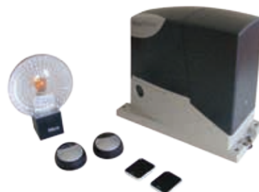
Kit NICE ROBUS 400 , moteur à coulissant autobloquant pour portail coulissant
