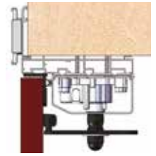
Coupe précadre et capot
