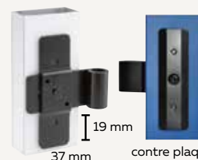
Équerre réglable EASY pour volets à cadre alu uniquement
