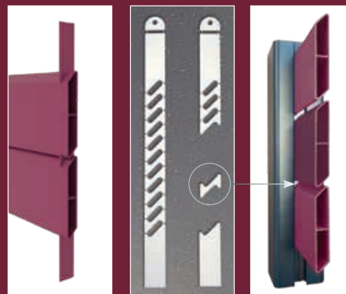
Intercalaires pour entre-lames
